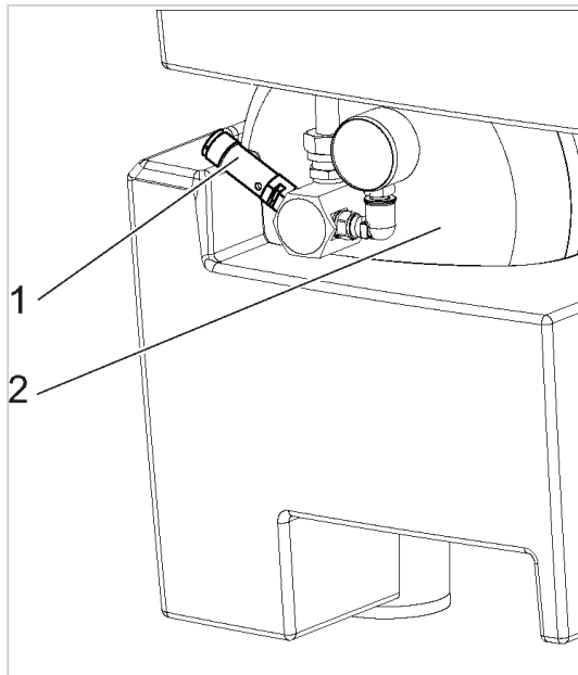
Abb. 20 Sicherheitsventil prüfen
