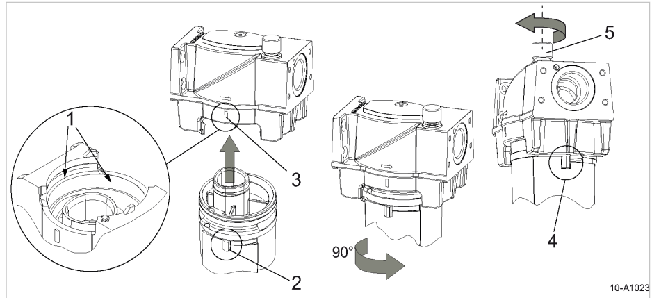
Abb. 7 Filterglocke montieren
