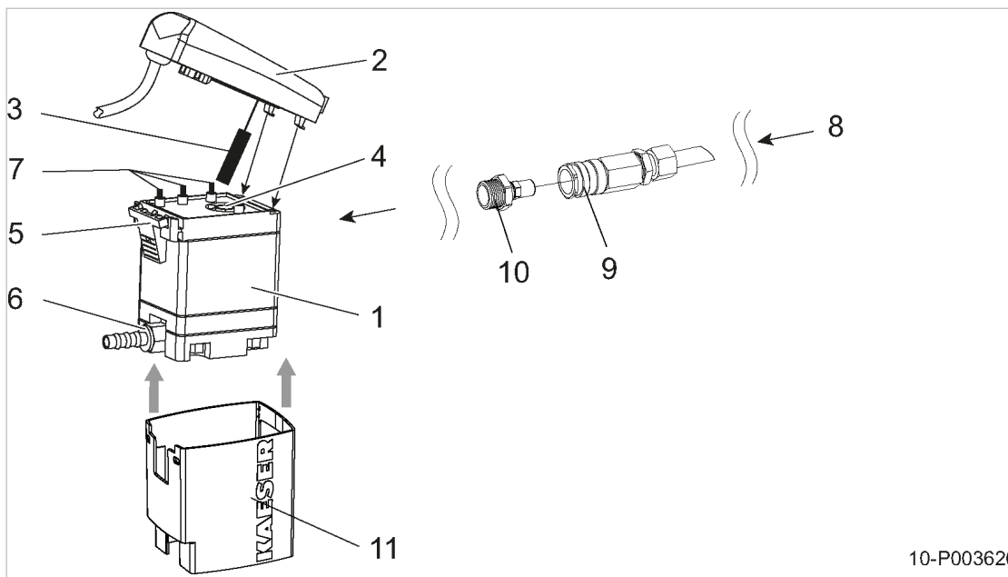
Abb. 27 Service-Unit wechseln
