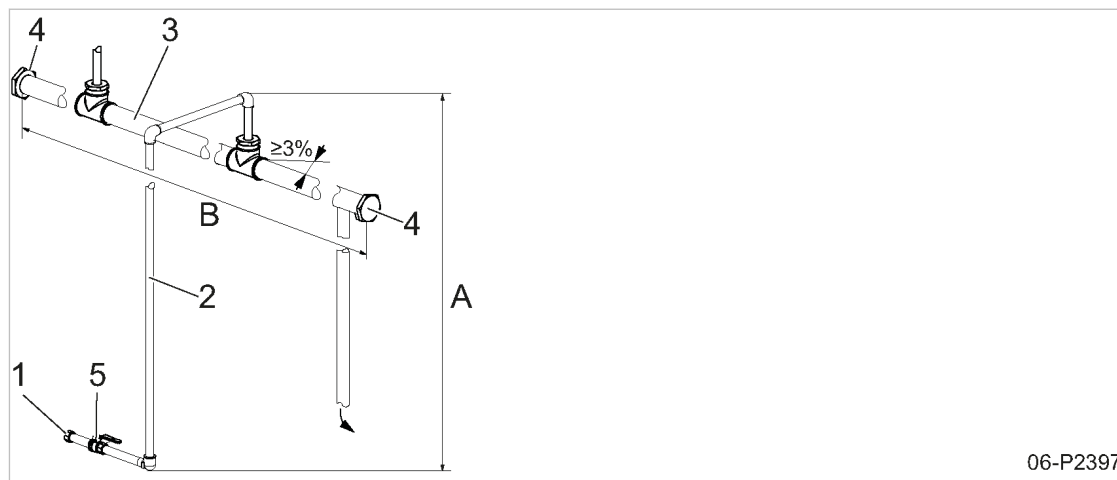
Abb. 13 Kondensatableiter anschließen
