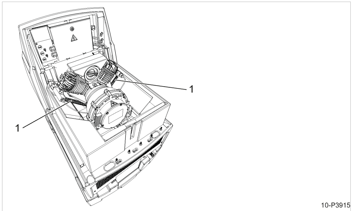
Abb. 22 Druckluftkühler
