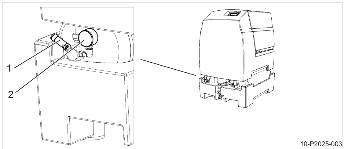
Abb. 21 Maschine entlüften
