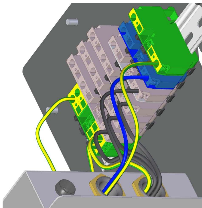
Bild 10: Zuleitungsanschluss
