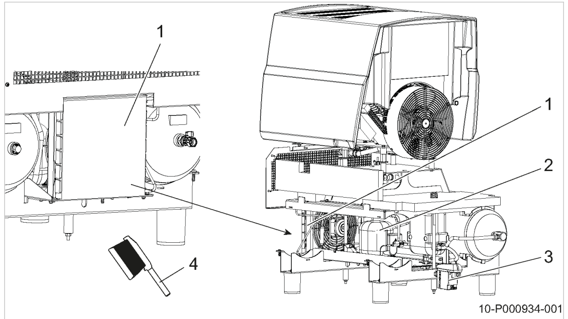
Abb. 25 Kältetrockner
