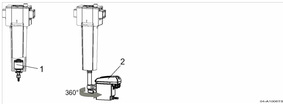
Abb. 3 Kondensatableiter
