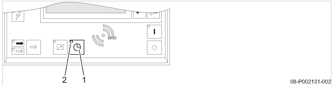
Abb. 16 Ein- und Ausschalten über die Zeitsteuerung
