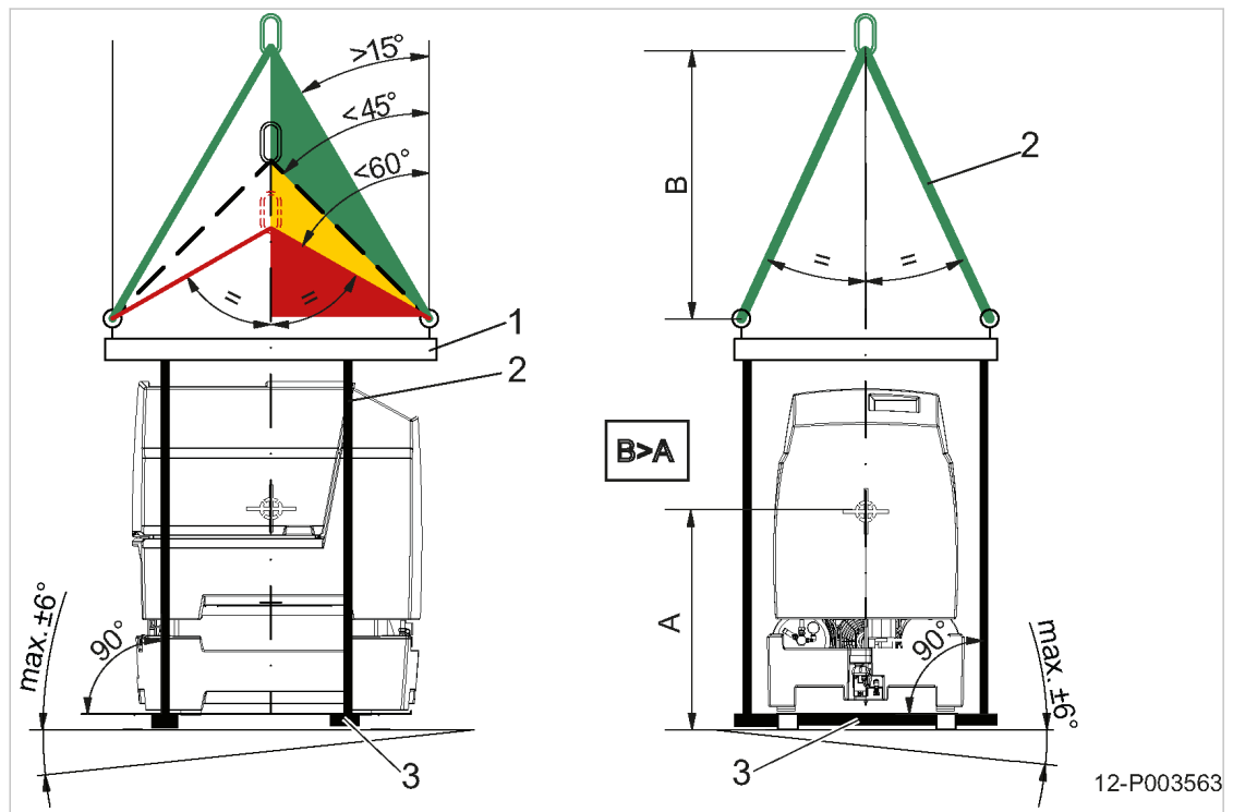
Abb. 29 Mit Kran transportieren
