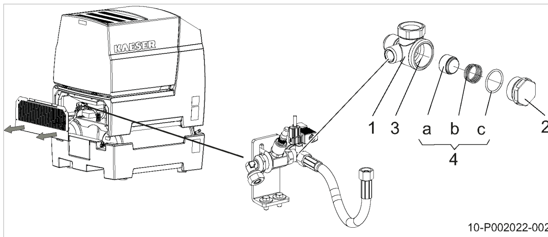
Abb. 23 Rückschlagventil reinigen
