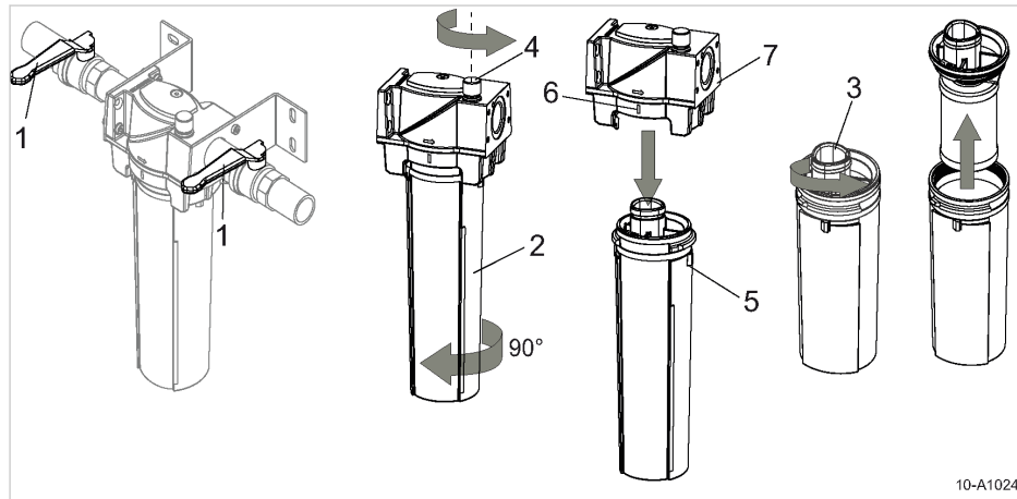
Abb. 5 Filterelement demontieren
