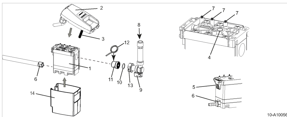
Abb. 10 Service-Unit wechseln
