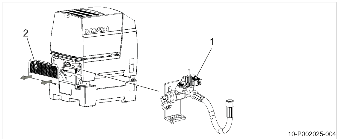
Abb. 24 Entlastungsventil ersetzen
