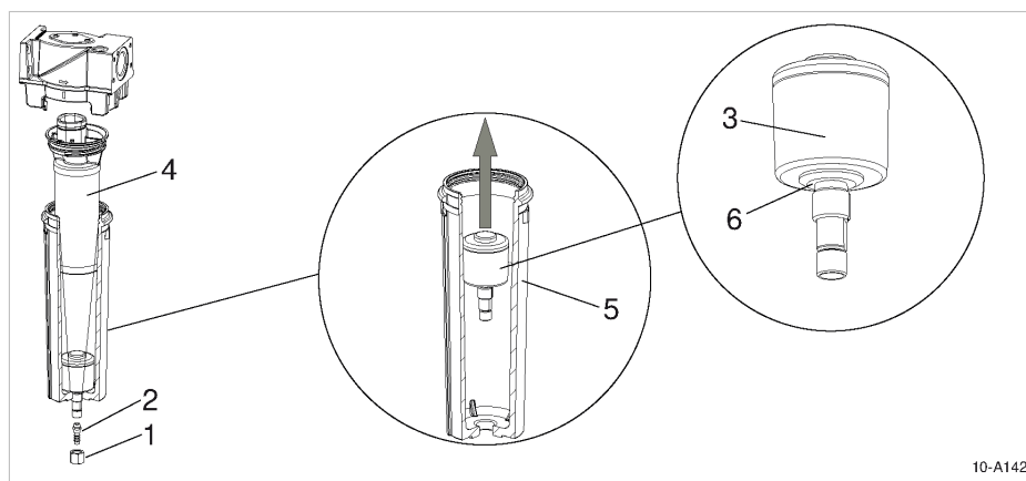
Abb. 11 Schwimmer ersetzen
