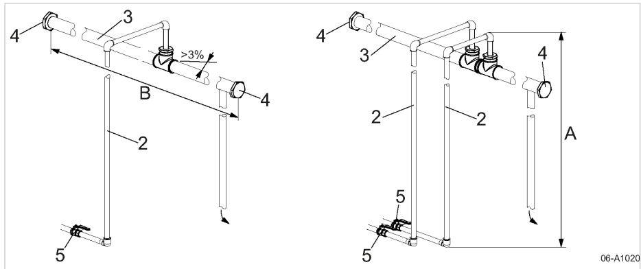
Abb. 4 Kondensatableiter anschließen
