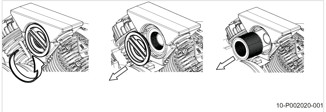
Abb. 18 Luftfilter ersetzen
