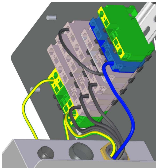
Bild 11: Zuleitungsanschluss
